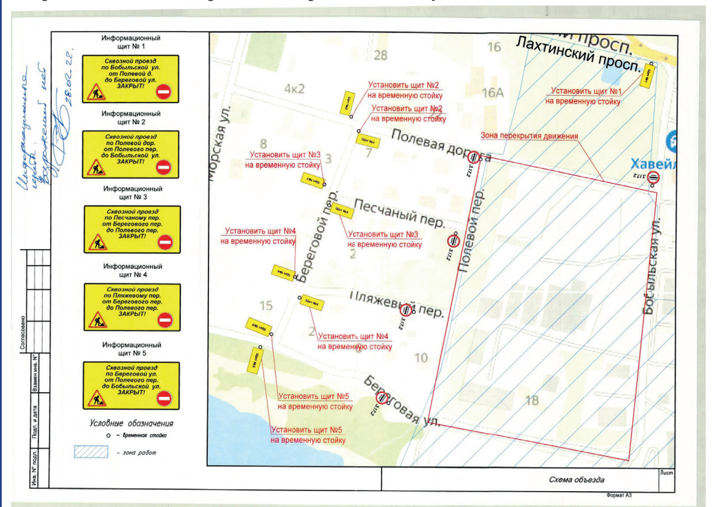
Временная схема объезда
